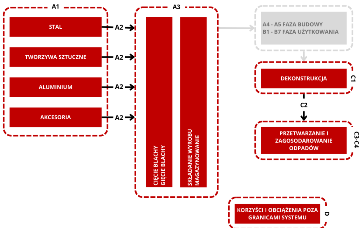
Rysunek 5.1: Granice systemu dla charakterystyki środowiskowej grzejników elektrycznych
